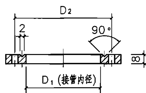
法兰A 3
