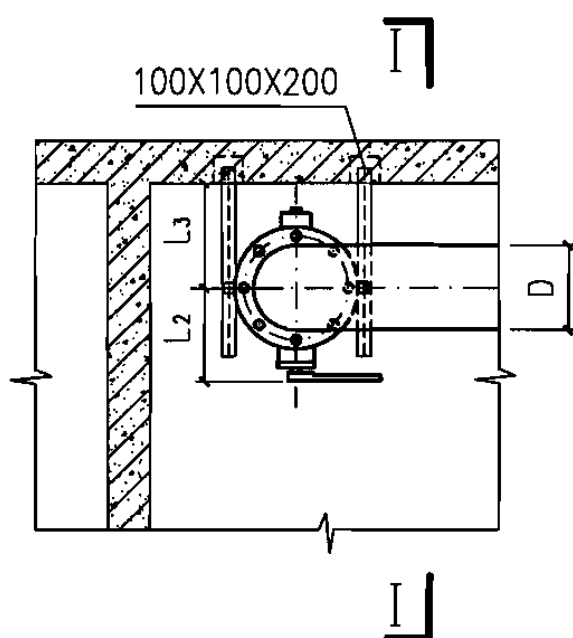
手动平面图
