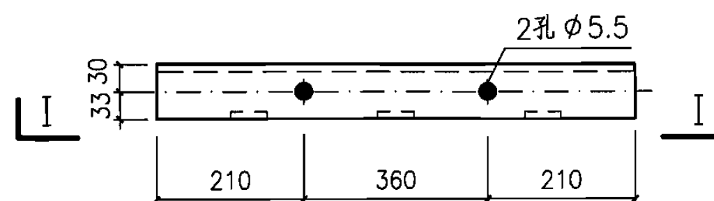
底架平面图
