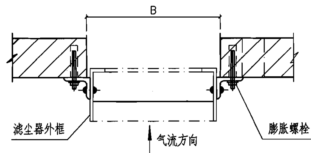
平面图
