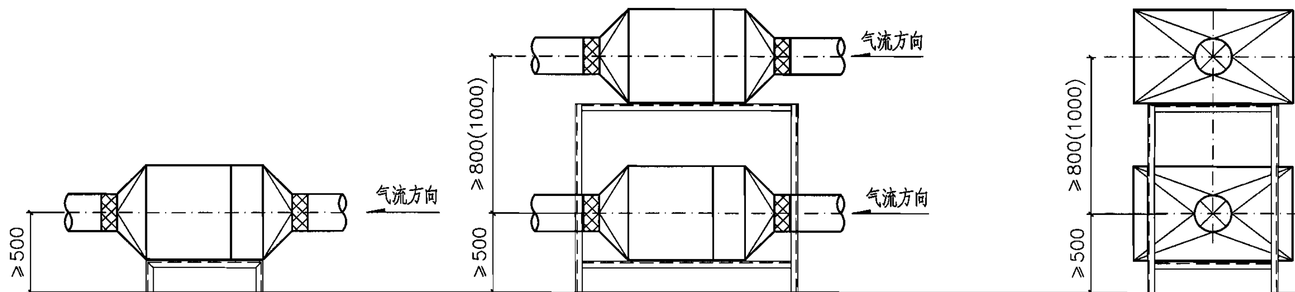
立面图(单)
