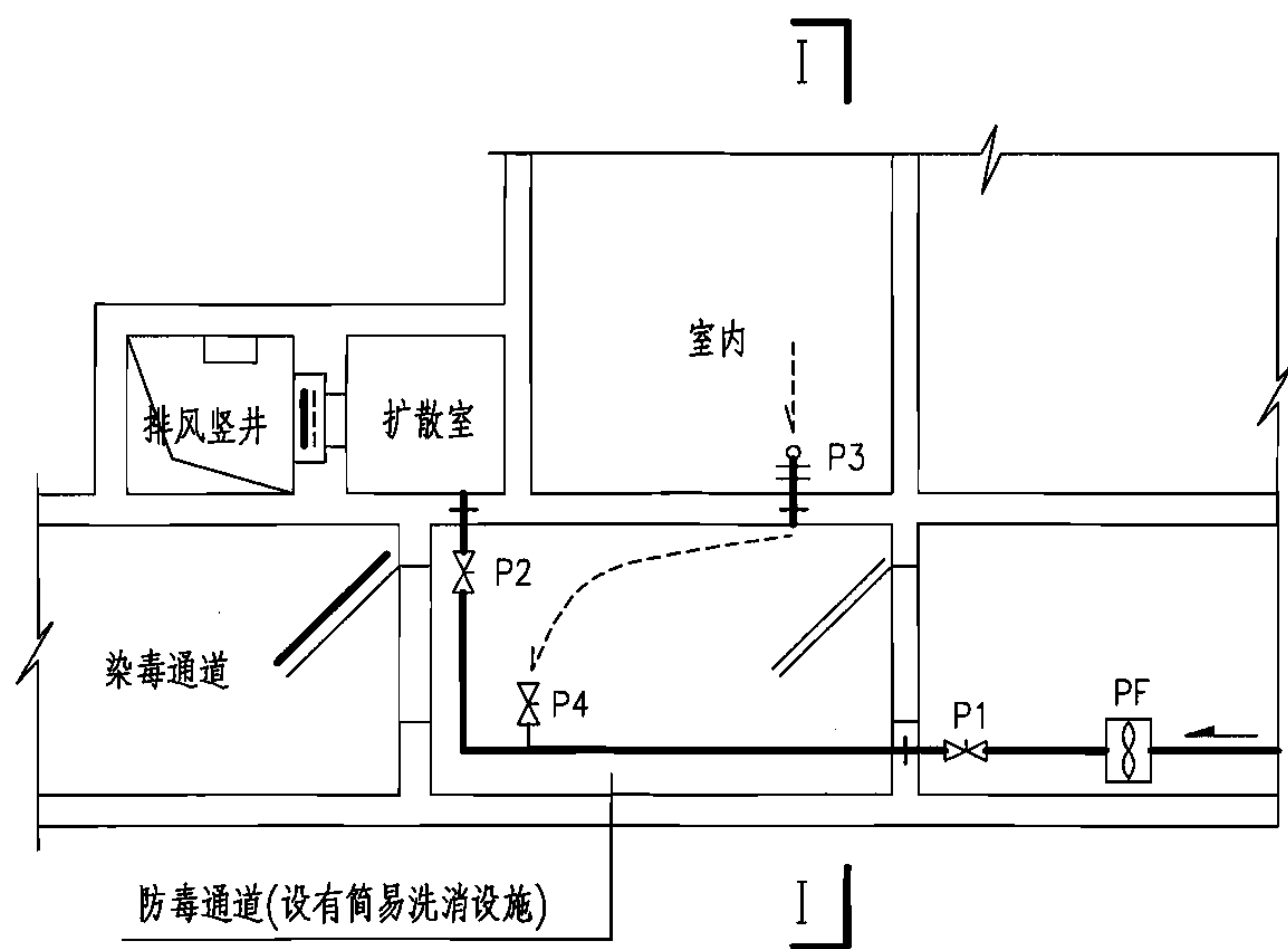
平面图
