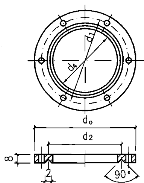
法兰A3
