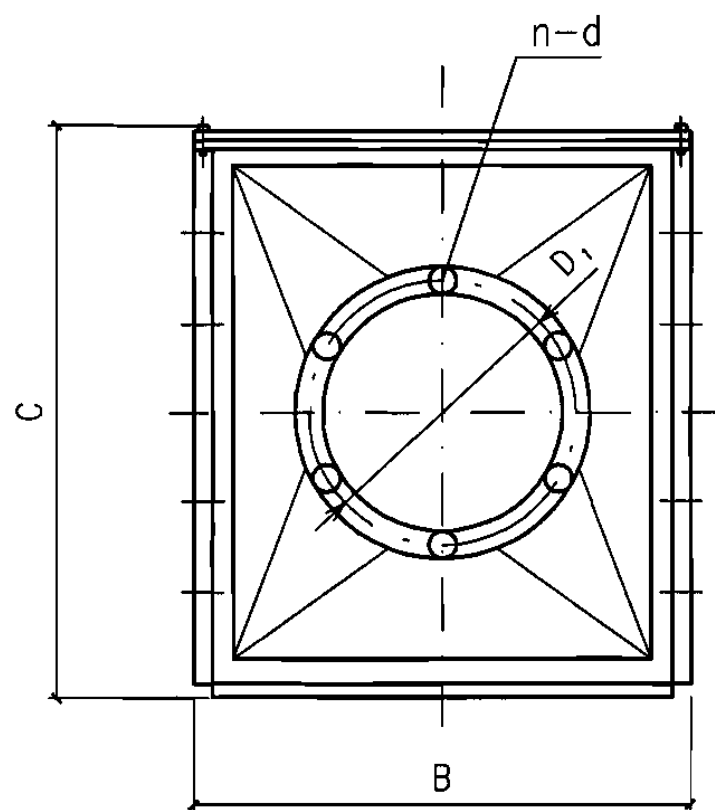
侧面图
