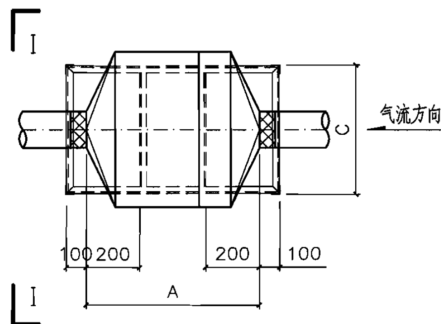
平面图(双)
