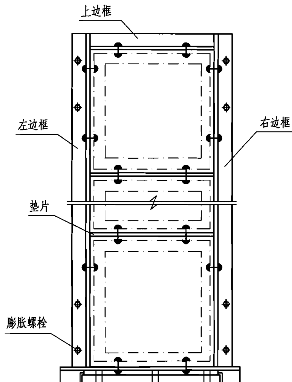
立面图
