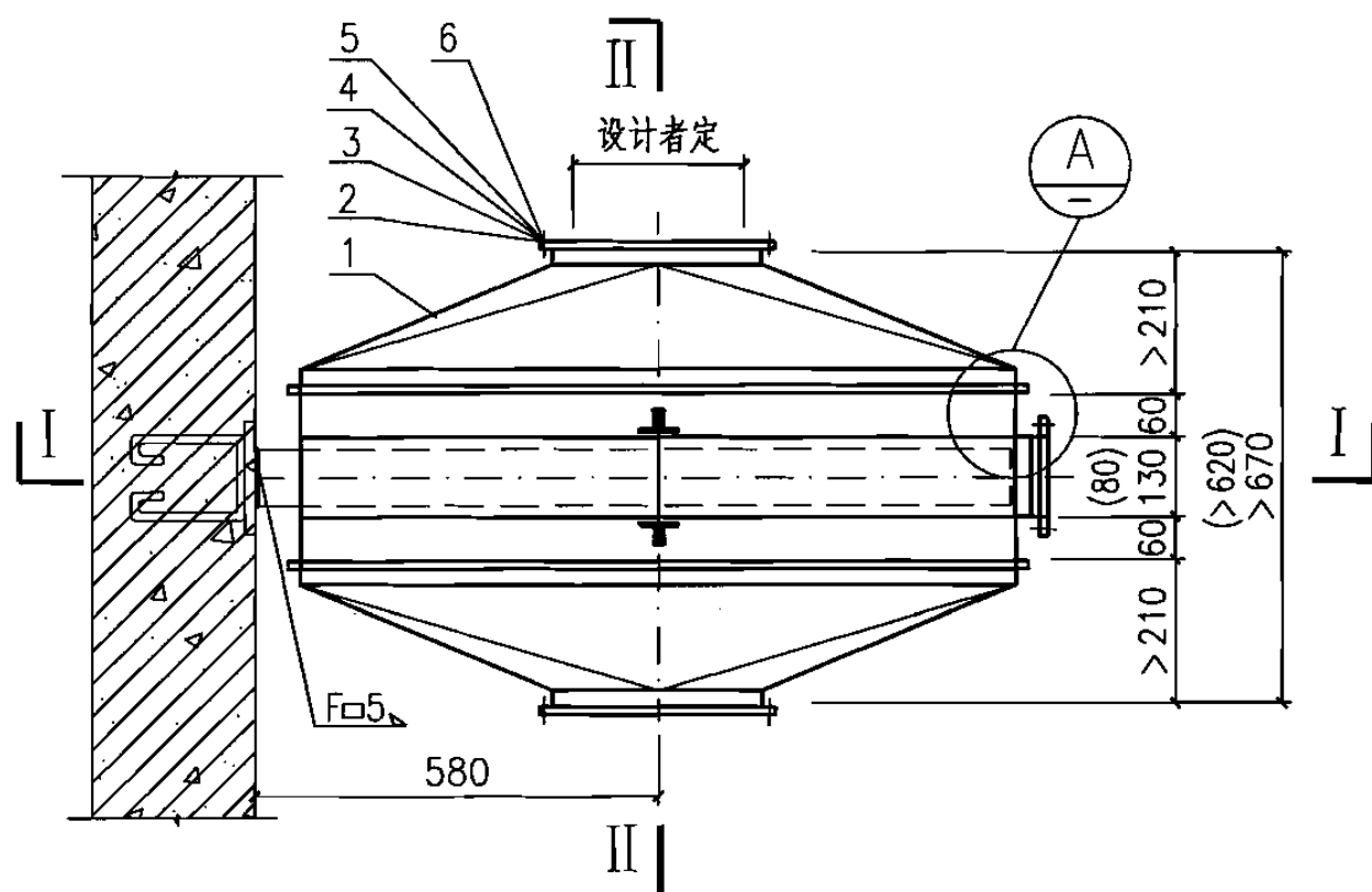
平面图
