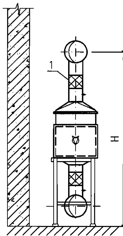
侧面图
