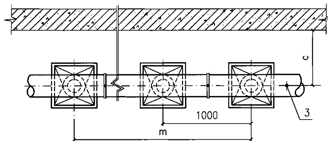
平面图
