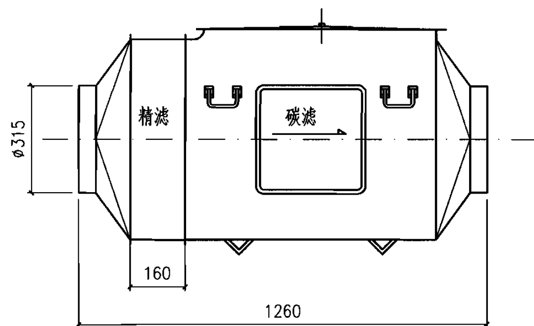
立面图
