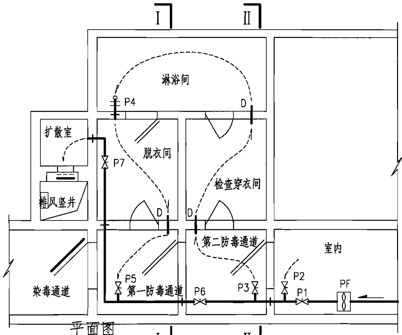
平面图
