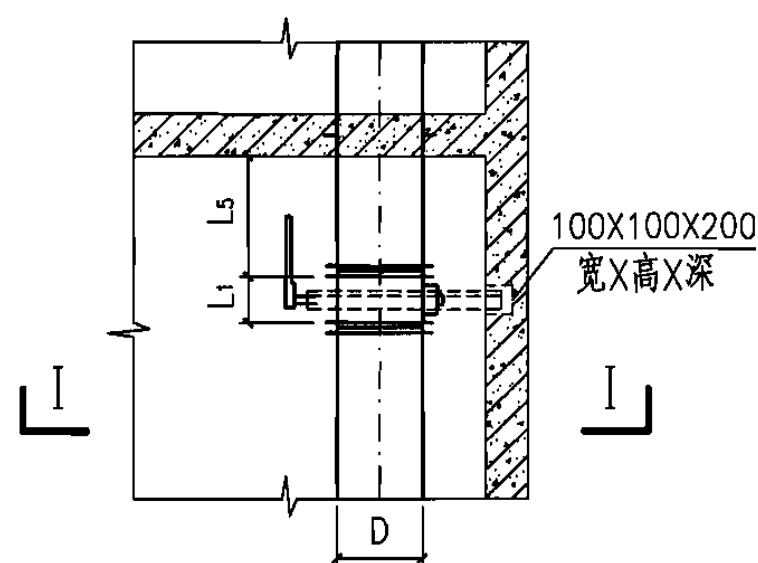
手动平面图
