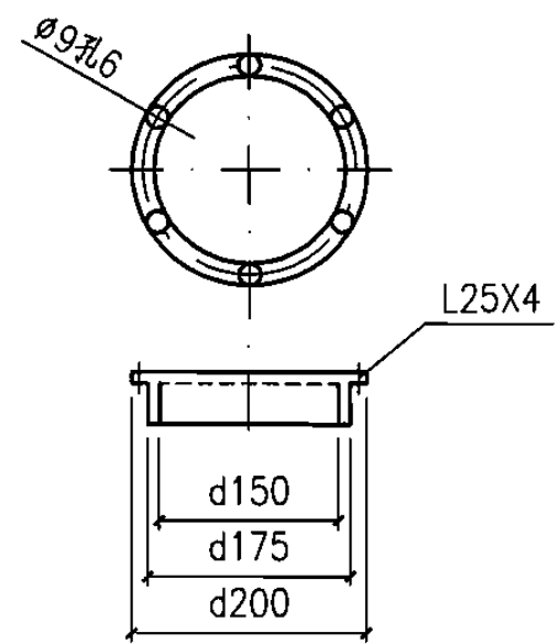
法兰平剖面图
